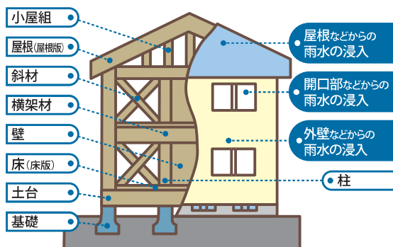
木造(在来軸組工法)の戸建住宅
